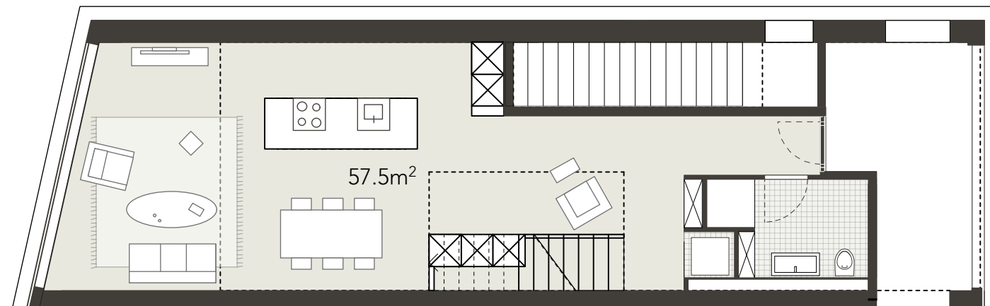
Zugangsgeschoss (1.OG)
